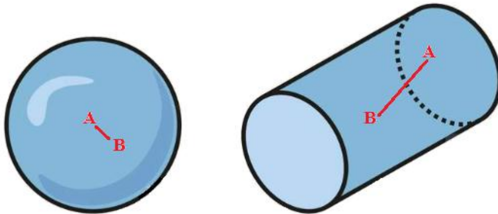
Fig. 1-6 - Se non vi è alcuna deformazione delle curvature le geodetiche energetiche coincidono con le geodetiche nel senso geometrico del termine.
