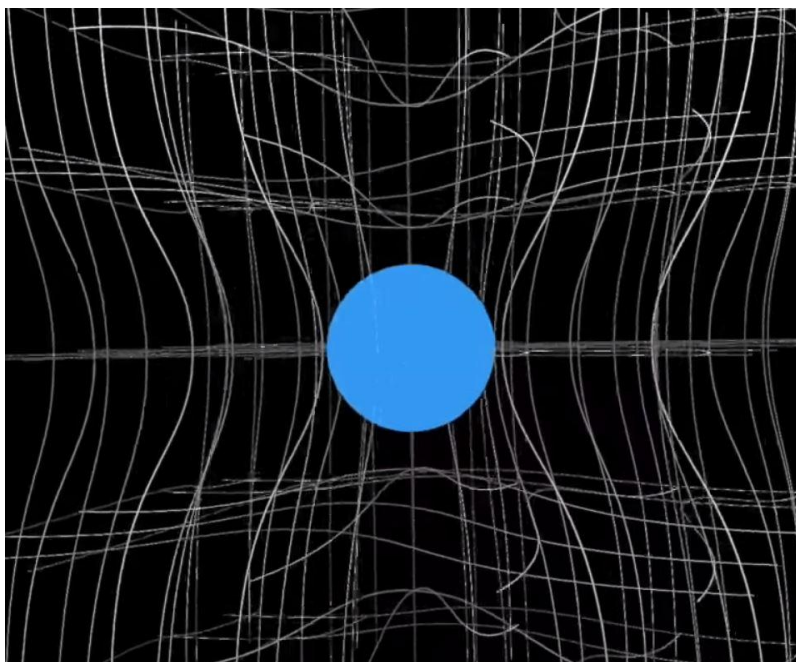
Fig. 1-3 – Un’altra divulgazione di come una “distorsione” spaziale determina la “forza” attrattiva della gravitazione. Fonte: https://www.youtube.com/watch?v=-m3SddsTSAY (accesso nel settembre 2021).
