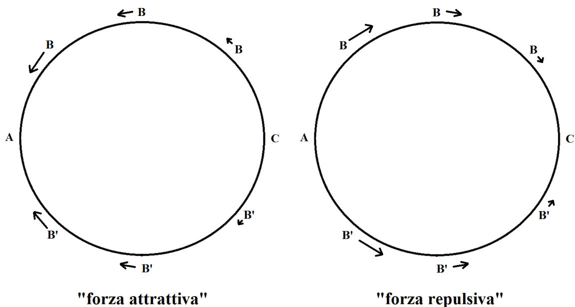
Fig. 1-14 – In C, che è agli antipodi di A (ovvero quando d_X = \pi \cdot R_X ), il valore della forza attrattiva (o repulsiva) deve essere necessariamente nullo. Se questo valore fosse diverso da 0, una “particella” in C dovrebbe andare contemporaneamente in due direzioni diverse, sia nel caso di una “forza attrattiva” (a sinistra) sia nel caso di una “forza repulsiva” (a destra).
