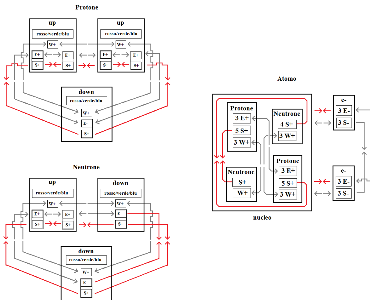
Fig. 2-2 - Modello 1, con una singola particella W+ nel quark up. Schemi di protone, neutrone e atomo. Parte delle attrazioni / repulsioni sono omesse per semplificare lo schema.
