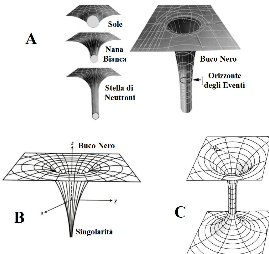
Fig. 3-4 - A e B: due rappresentazioni di un buco nero e della singolarità che sarebbe al suo centro; C: un ipotetico tunnel tra due parti dello spaziotempo causato da una singolarità.
