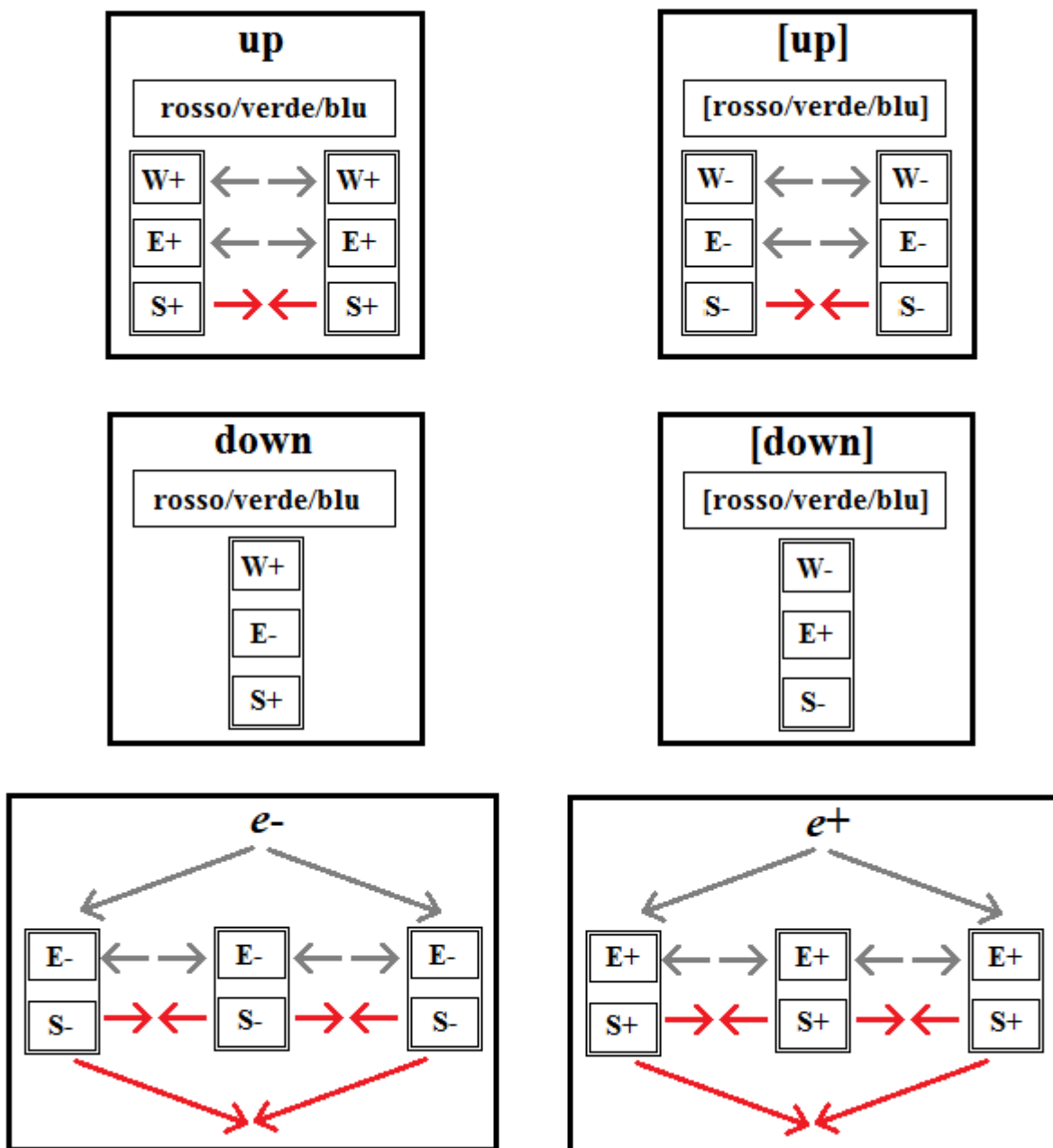
Fig. 2-5 - Modello 2, con due particelle W^+ nel quark up. Schemi dei quark up, [up], down, [down], dell'elettrone ( e^- ) e del positrone ( e^+ ).
