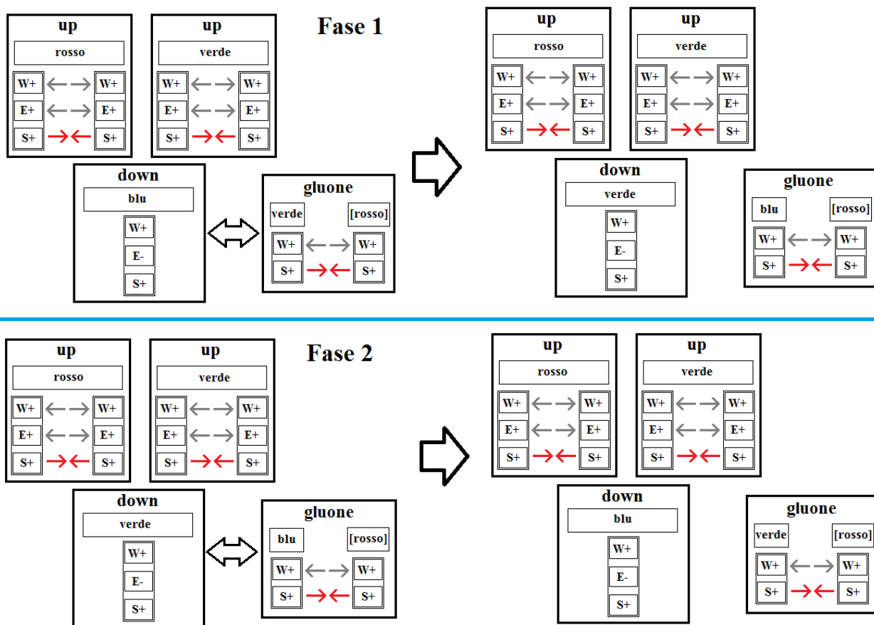
Fig. 2-9 – Un esempio di ciclo di interazione, in due fasi, tra un quark down e due gluoni (in un protone). Nella prima fase, il colore del quark down cambia da blu a verde per interazione con un gluone, ma poiché due quark hanno ora lo stesso colore (verde), il complesso è instabile. Nella seconda fase, il quark down ritorna al colore blu e la tripletta di quark è di nuovo stabile.
