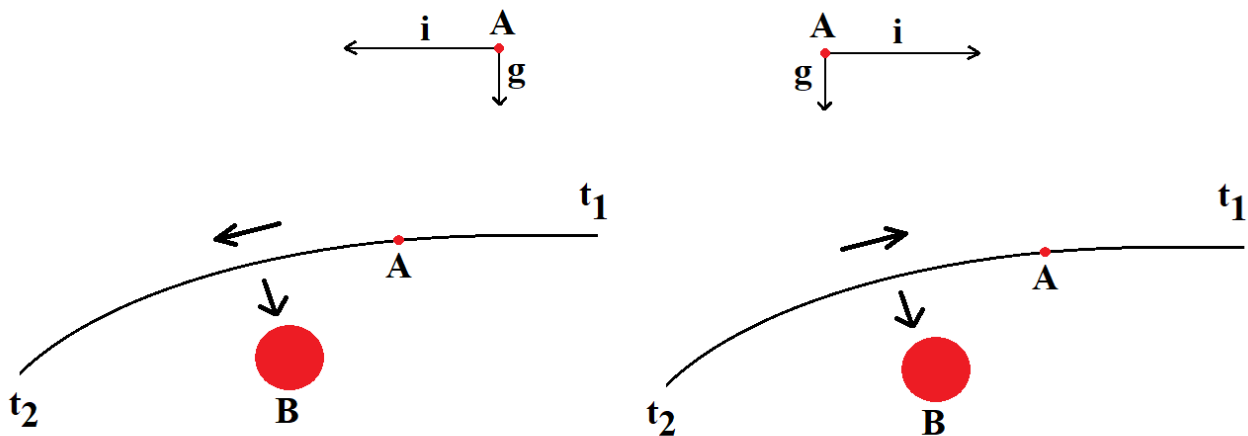
Fig. 3-10 – A sinistra: il corpo A mostra due movimenti: il moto inerziale (i) e lo spostamento (g) verso il corpo B causato dalla “forza” gravitazionale. A destra: invertendo le coordinate temporali di riferimento, il moto (i) si inverte mentre lo spostamento (g) non si inverte.
