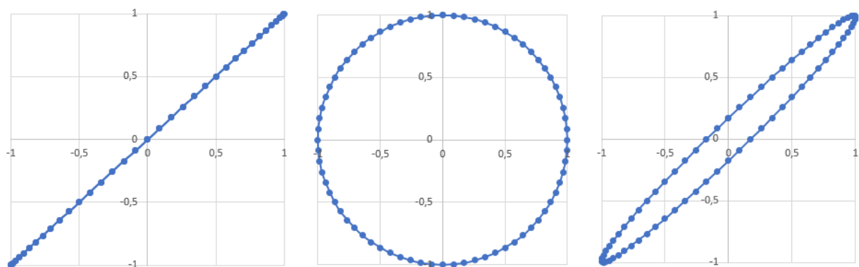
Fig. 1-9 – Una doppia oscillazione vista di fronte. Sono riportati i valori del seno di un punto sulle due curve. A sinistra: le due oscillazioni sono sincrone; al centro: le due oscillazioni sono sfasate di 90^\circ ; a destra: le due oscillazioni sono sfasate di 10^\circ .
