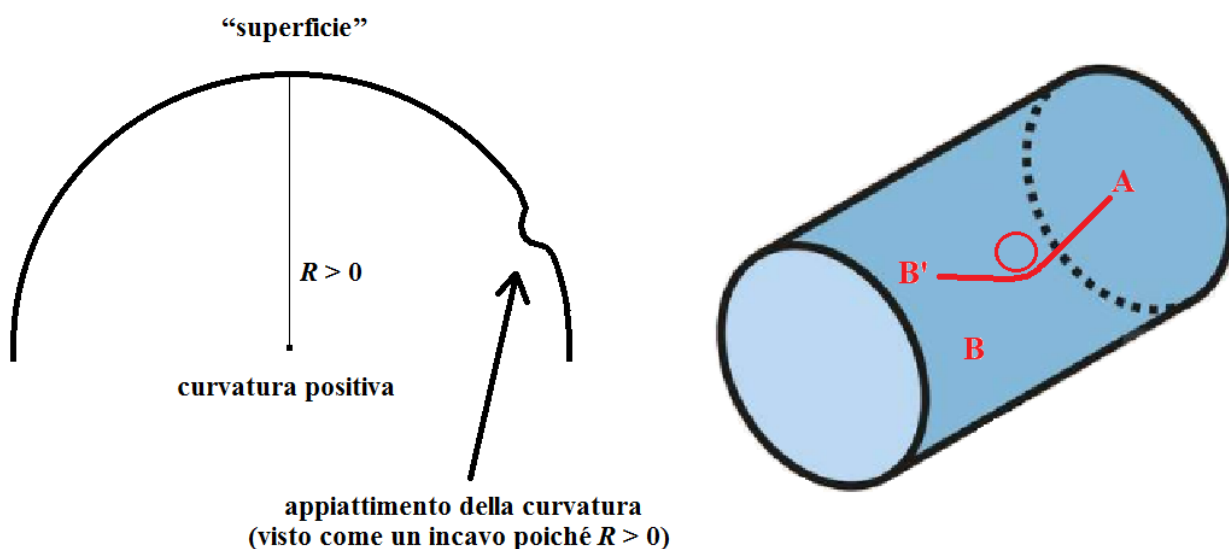
Fig. 1-7 – In questa figura come in quella successiva, per meglio evidenziarli graficamente, gli appiattimenti sono raffigurati come marcati incavi o come marcate sporgenze. In realtà dovrebbero essere raffigurati come tratti della circonferenza con minore curvatura, ma in tal caso sarebbero invisibili o poco visibili. L'appiattimento determina una modifica della geodetica energetica A-B avvicinandola all'appiattimento e così deviandola verso B'.
