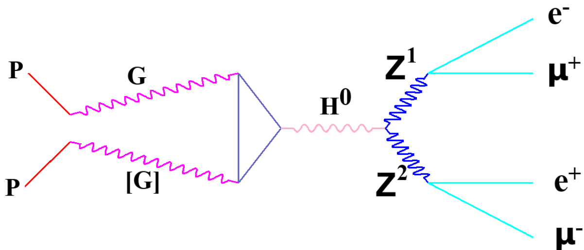
Fig. 2-12 – Formazione e decadimento del bosone di Higgs.
