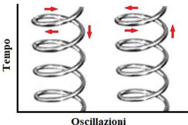
Fig. 1-11 – A destra: il moto dell’apice di una doppia oscillazione per una “particella”; a sinistra: lo stesso per una “antiparticella”.
