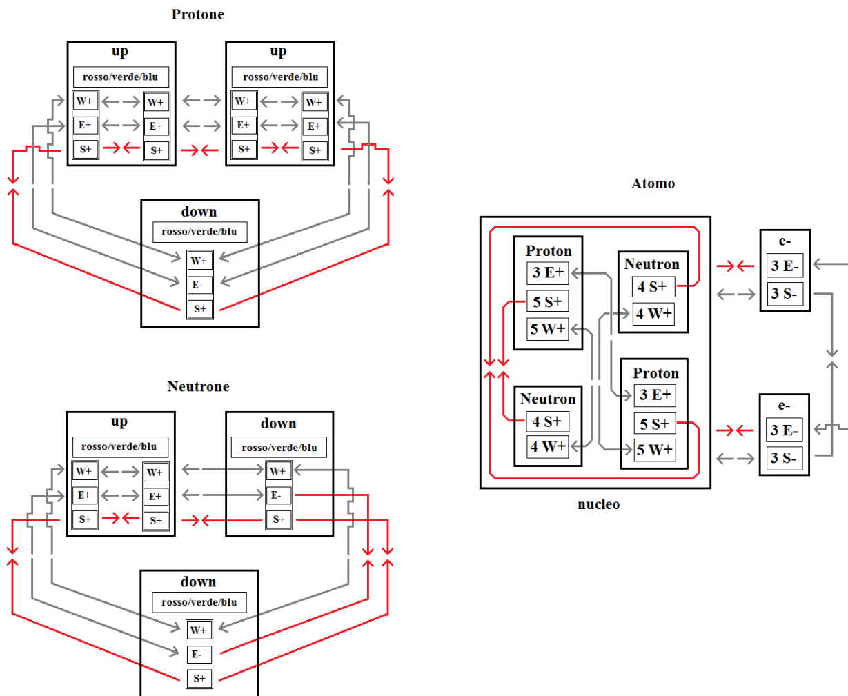
Fig. 2-4 - Modello 2, con due particelle W^+ nel quark up. Schemi di protone, neutrone e atomo. Parte delle attrazioni / repulsioni sono omesse per semplificare lo schema.
