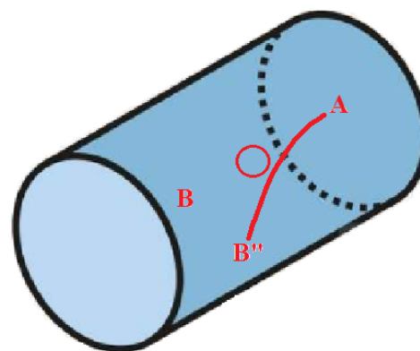
Fig. 1-8 - In questo caso l'appiattimento è come un rilievo (un picco di energia) e la geodetica energetica A-B si allontana dall'appiattimento deviando così verso B".
