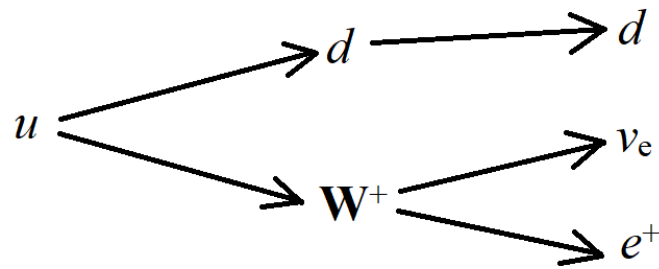
Fig. 2-11 - Reazione 1 [Veltman 2003, p. 100] + Reazione 5 [Rohlf 1994]
