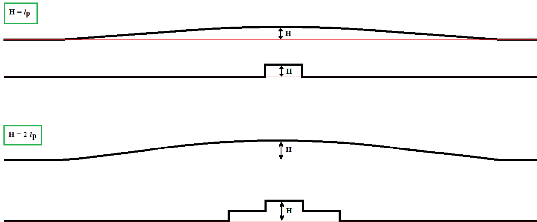
Fig. 1-16 – Sopra, un’onda con ampiezza massima ( H ) pari a una lunghezza di Planck ( l_p ). Se le dimensioni in cui si allarga l’onda nelle direzioni trasversali non fossero infinitamente divisibili, l’ampiezza dovrebbe passare da H a 0 con un unico gradino di altezza l_p . Sotto, un’onda con H = 2 l_p . In questo secondo caso l’onda dovrebbe passare da H a 0 con due gradini di altezza l_p .
