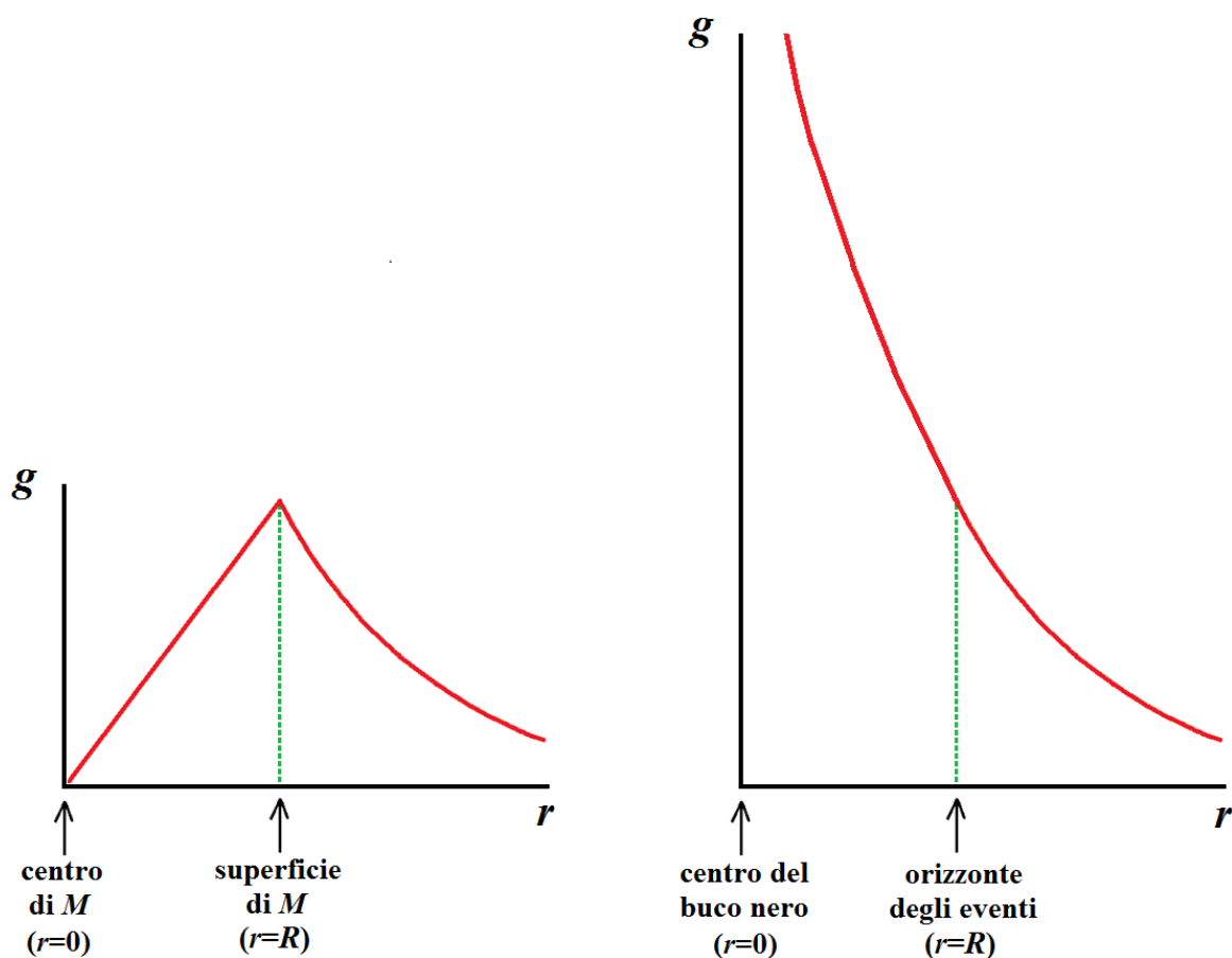
Fig. 3-5 – A sinistra: variazione della gravità in funzione della distanza r dal centro di M per qualsiasi massa che non sia un buco nero. A destra: variazione ipotetica della gravità in funzione di r per un buco nero (secondo l'interpretazione corrente).
