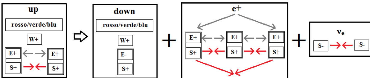
Fig. 2-6 - Interpretazione del decadimento beta- e del decadimento beta+ secondo il modello 1.
