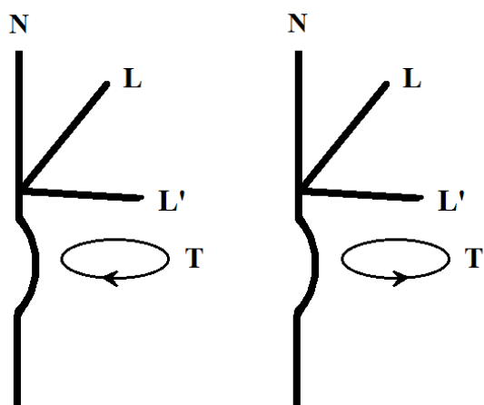
Fig. 3-6 - A sinistra, un segmento della dimensione Spaziale o Newtoniana N , visto dall'alto dell'immagine, ruota in senso orario attorno alla dimensione Spaziale N nelle dimensioni L e L' , mentre a destra ruota in senso antiorario. I due tipi di rotazioni sono definiti arbitrariamente rispettivamente come positivi e negativi. La dimensione Spaziale N è una dimensione curva, ma la curvatura è troppo piccola per la scala dell'immagine. Inoltre, la curva del segmento rotante è stata marcatamente esagerata per renderla visibile. L e L' sono due dimensioni con curvatura nulla o quasi nulla.
