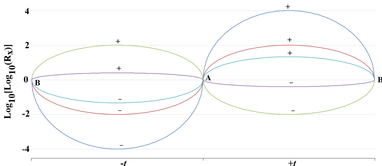
Fig. 4-3 – Come sviluppo dell'ipotesi anzidetta, ciascuna dimensione dopo aver raggiunto un raggio massimo ( r_x oppure -r_x ), riduce il valore assoluto del suo raggio fino al suo azzeramento in un punto B che è unico per le due direzioni “meta-temporali”. La rappresentazione in piano delle n dimensioni dovrebbe intendersi come avvolta sulla superficie di un cilindro con A e B in posizioni opposte.
