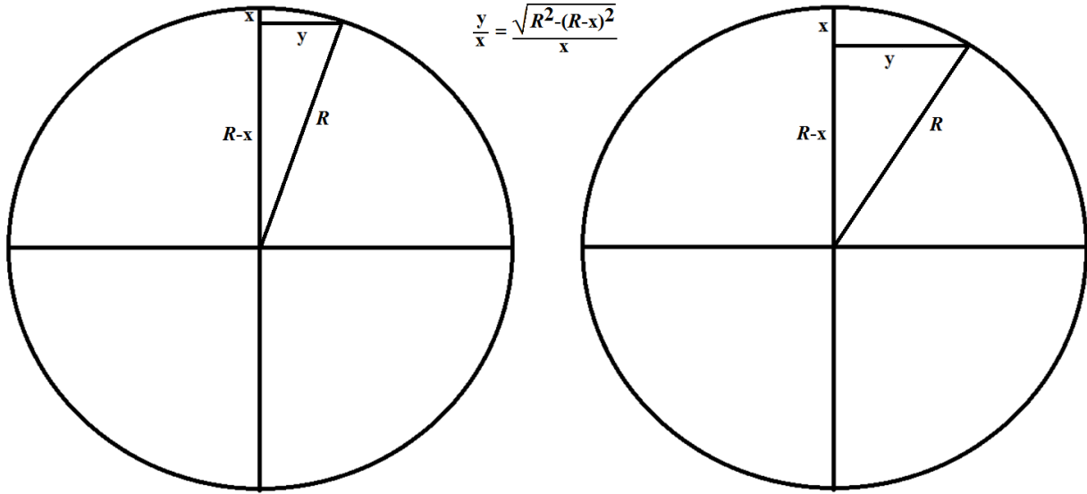
Fig. 3-2 - Definendo la misura dell'appiattimento come il rapporto y/x , questo rapporto è massimo quando x è il minimo possibile.
