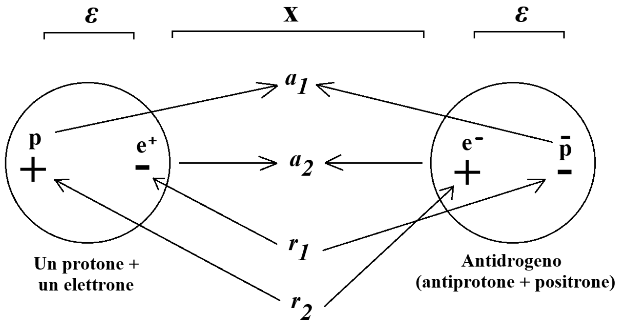
Fig. A-1 – Attrazioni e repulsioni elettriche fra atomi di idrogeno e di antidrogeno.
