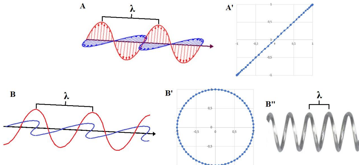
Fig. 3-7 – A: Schema di una doppia oscillazione (o onda) sincrona; A': Il movimento di un punto dell'onda rappresentato in A visto frontalmente; B: Schema di una doppia oscillazione asincrona con sfasamento fra le due oscillazioni di 90^\circ ; B': Il movimento di un punto (P) dell'onda rappresentato in B visto frontalmente. Il valore di r (raggio del movimento di P visto frontalmente) è pari a \lambda/4 ; B'': Il movimento schematizzato di P in una vista tridimensionale è analogo a quello della spira di una molla.
