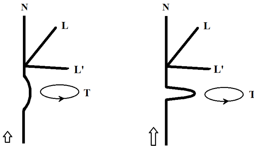
Fig. 3-9 - A sinistra, un segmento di dimensione N ruota mediante una doppia oscillazione attorno all'asse di N nelle dimensioni L e L' , che sono non curve o con minima curvatura. La curvatura della dimensione N è molto lieve per la scala dell'immagine e non può essere visibile, mentre la curva del segmento rotante è stata notevolmente esagerata. L'appiattimento determinato dalla rotazione e definito come "particella", si muove nella direzione indicata dalla freccia. A destra, mentre la particella aumenta la sua velocità (indicata dalla freccia più grande), assume quanti delle dimensioni N e T (indicati dal rigonfiamento crescente). L'assunzione di quanti delle due dimensioni significa per la particella un accorciamento della sua lunghezza secondo la direzione di N , un aumento della sua massa/energia, e un rallentamento del passare del tempo rispetto ad altre particelle con velocità minore.
