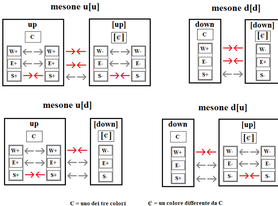
Fig. 2-10 – Schema dei quattro possibili mesoni considerando solo i quark u, d, e i relativi antiquark,
