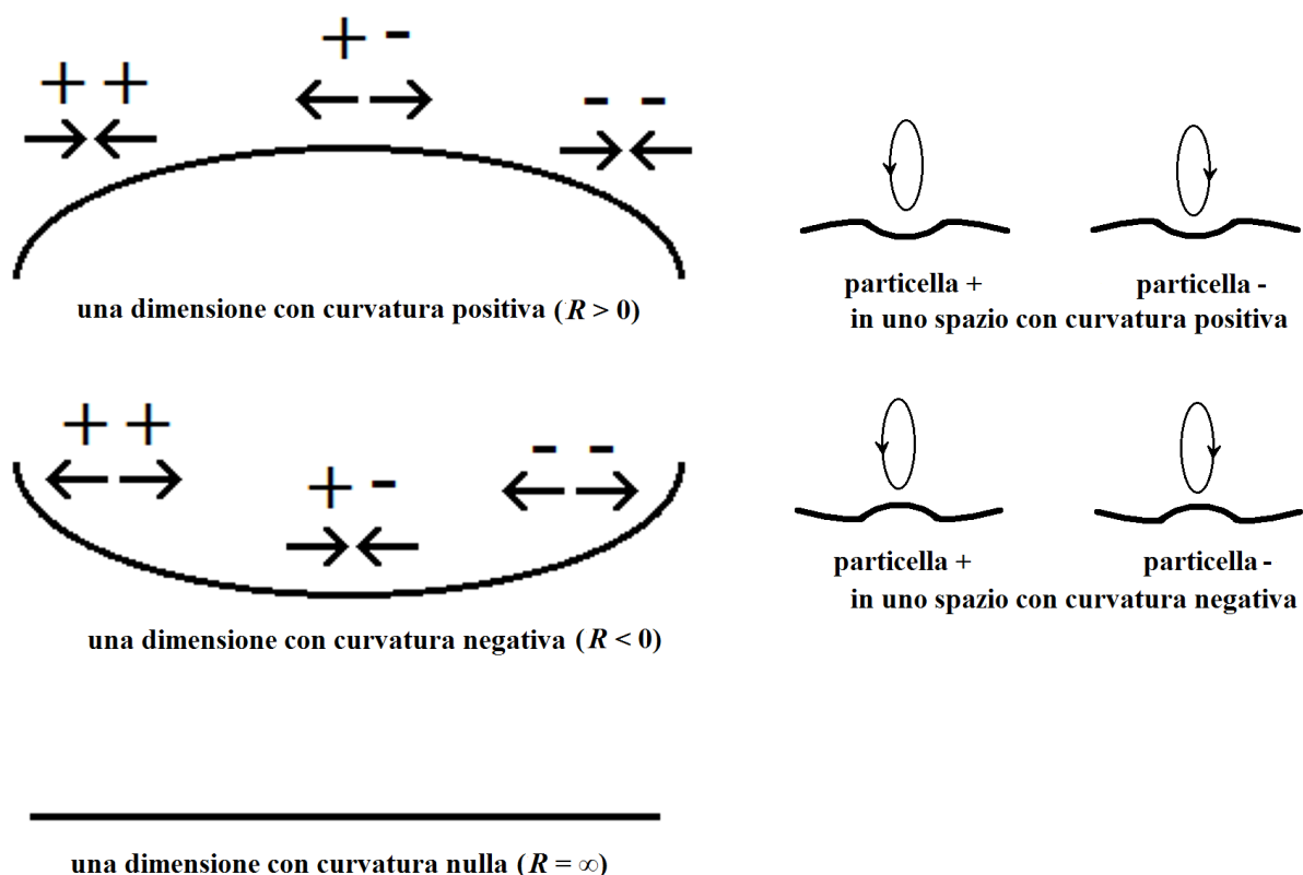
Fig. 1-12 - I tre possibili tipi di dimensioni. Le “particelle” sono rappresentate con il segno “+” o con il segno “-” a seconda che abbiano rotazione oraria o antioraria. Le “forze”, “attrattive” o “repulsive”, sono rappresentate rispettivamente da frecce convergenti o divergenti.
