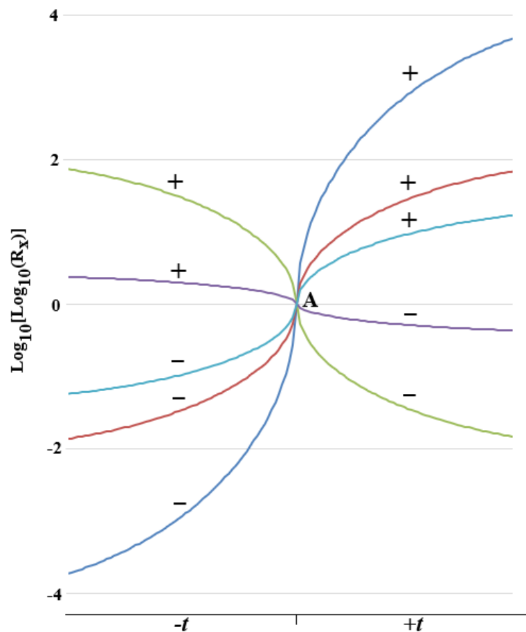
Fig. 4-2 – L'ipotesi prospettata in queste pagine: a partire da un punto A, in direzioni “meta-temporali” opposte, si espandono simmetricamente n dimensioni con curvatura opposta. E' da notare che l'immagine prospettata, per esigenze grafiche, riporta in un solo piano il progressivo aumento dei raggi. Comunque, le suddette dimensioni debbono essere intese come tutte ortogonali (o quasi ortogonali) fra di loro, il che per più dimensioni non è rappresentabile in una immagine. Inoltre, per motivi grafici, la scala dei raggi delle dimensioni è in \text{Log}_{10}[\text{Log}_{10}(R_x)] .
