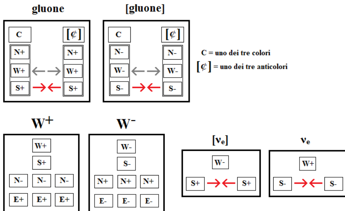
Fig. 2-14 - Possibili appiattimenti delle dimensioni Newtoniane (Spaziali) e di altre dimensioni nei gluoni, e nelle particelle W^+ e W^- (da non confondere con gli appiattimenti nella dimensione Debole ( W ), indicati dai simboli W^+ e W^- ). I gluoni sono abitualmente descritti come aventi massa zero. Il neutrino elettronico e l'antineutrino non devono avere alcun appiattimento nelle dimensioni newtoniane per spiegare la loro massa molto bassa o nulla.
