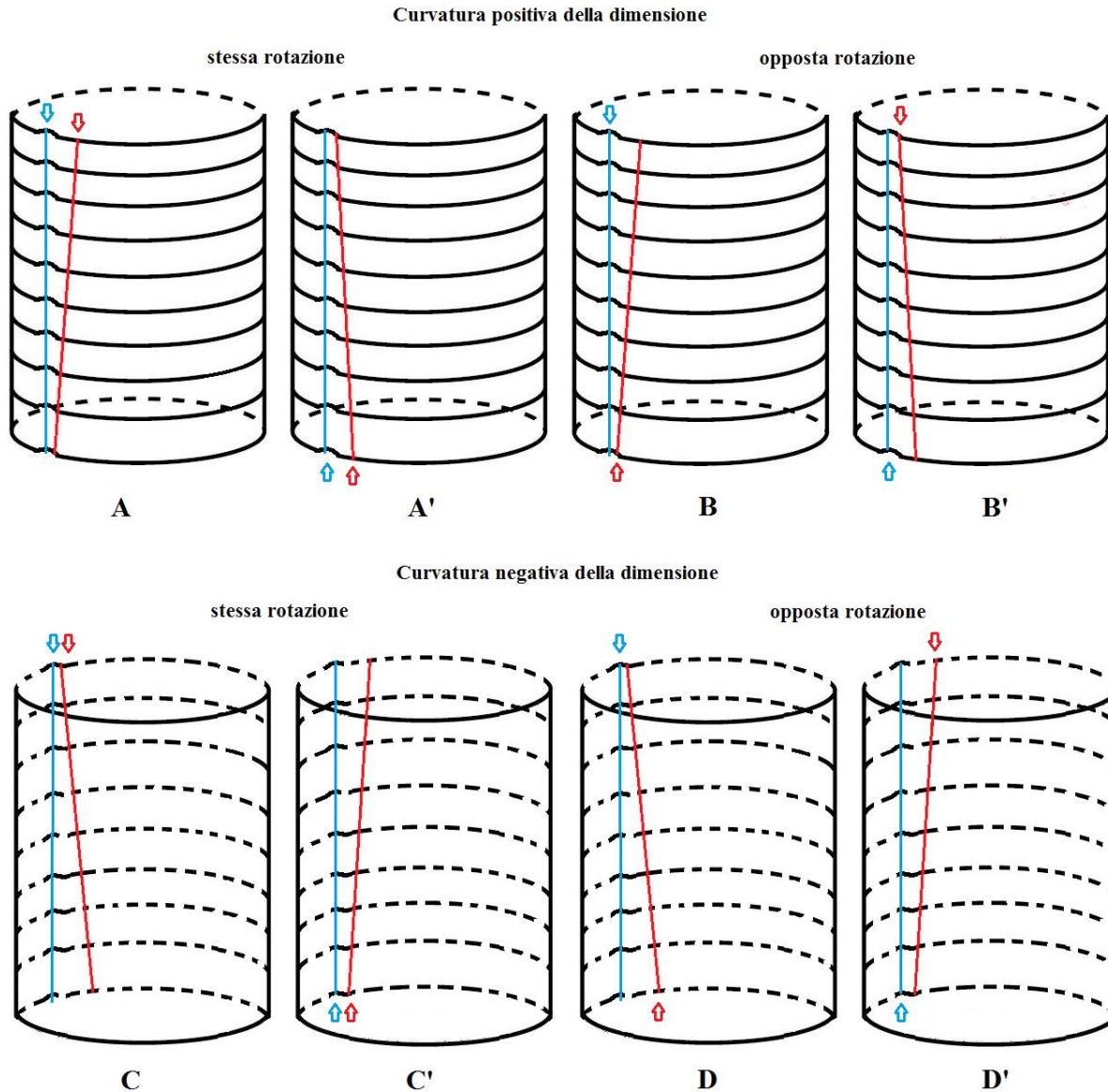
Fig. 1-10 - Schema degli spostamenti degli appiattimenti a seconda funzione della curvatura dello spazio e del valore (positivo o negativo) delle rotazioni. L'appiattimento maggiore è indicato da una freccia azzurra, mentre l'appiattimento minore da una freccia rossa. Lo spostamento dell'appiattimento maggiore è molto piccolo (non rappresentato) ed è indicato da una linea azzurra mentre quello dell'appiattimento minore è indicato da una linea rossa. Nella parte superiore una dimensione ha curvatura positiva mentre l'altra ha curvatura nulla; nella parte inferiore una dimensione ha curvatura negativa mentre l'altra ha curvatura nulla; a sinistra (A, A', C, C') le rotazioni hanno gli stessi valori; a destra (B, B', D, D') le rotazioni hanno valori opposti. Per una migliore leggibilità dello schema, ogni appiattimento è fortemente esagerato diventando un marcato incavo o rigonfiamento.
