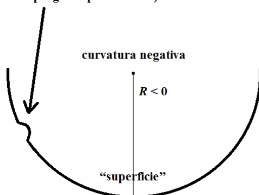
Fig. 1-8 - In questo caso l'appiattimento è come un rilievo (un picco di energia) e la geodetica energetica A-B si allontana dall'appiattimento deviando così verso B".
