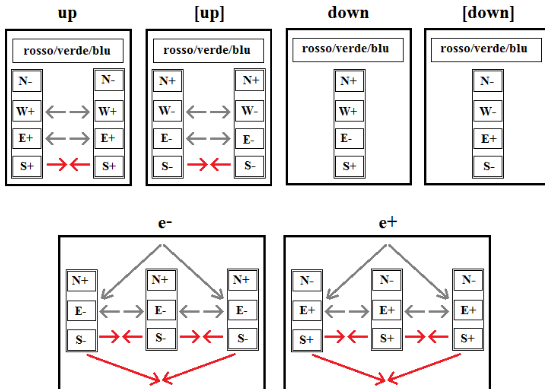
Fig. 2-13 – Possibili appiattimenti delle dimensioni Newtoniane (Spaziali) e di altre dimensioni nei quark u , d ; negli antiquark [u] , [d] , nell'elettrone ( e^- ) e nel positrone ( e^+ ).
