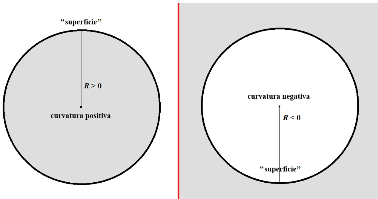
Fig. 1-5 - Una rappresentazione schematica di una dimensione con curvatura positiva (a sinistra) e di una dimensione con curvatura negativa (a destra).
