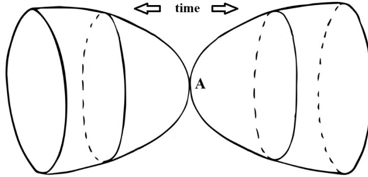
Fig. 4-1 – L'idea generale del Janus universe : a partire da un punto A si ha una espansione delle dimensioni in due direzioni temporali opposte.
