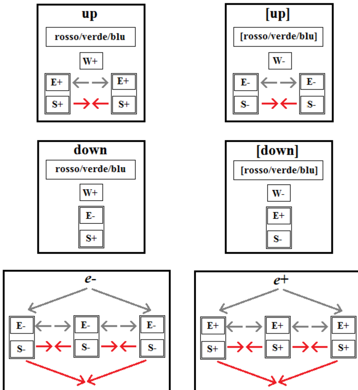
Fig. 2-3 - Modello 1, con una singola particella W^+ nel quark up. Schemi dei quark up, [up], down, [down], dell'elettrone ( e^- ) e del positrone ( e^+ ). I raggruppamenti di più particelle che sono comunemente indicati come antiparticelle sono racchiusi tra parentesi quadre. Ad esempio: anti-up = [up]. Per uniformità di scrittura, l'elettrone si dovrebbe indicare con e ed il positrone con [e] in alternativa alle abituali scritture e^- e e^+ .
