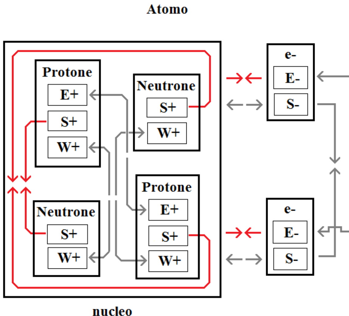
Fig. 2-1 - Schema generale della struttura atomica come ipotizzata. E+ ed E- = particella e antiparticella della dimensione Elettrica (E); S+ e S- = particella e antiparticella della dimensione Forte ("Strong", S); W+ e W- = particella e antiparticella della dimensione Debole ("Weak", W). Parte delle attrazioni / repulsioni sono omesse per semplificare lo schema.
