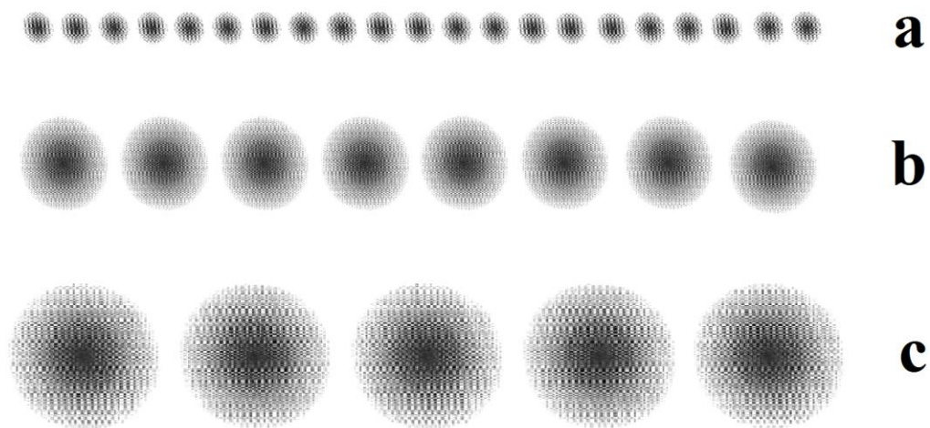
Fig. 3-8 – Tre serie di onde elettromagnetiche (fotoni) che si muovono nello spazio, con energia che decresce andando dall’alto (frequenza maggiore, lunghezza d’onda minore) verso il basso (frequenza minore, lunghezza d’onda maggiore).
