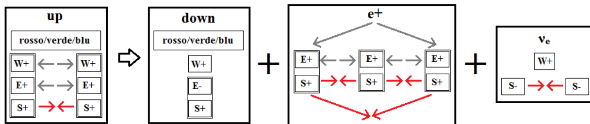
Fig. 2-7 - Interpretazione del decadimento beta- e del decadimento beta+ secondo il modello 2.
