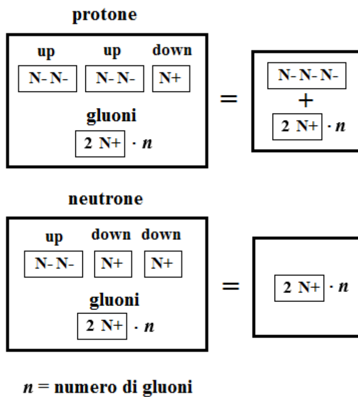
Fig. 2-15 - Possibili appiattimenti delle dimensioni Newtoniane (o Spaziali; appiattimenti per altre dimensioni non indicate) nel protone e nel neutrone.
